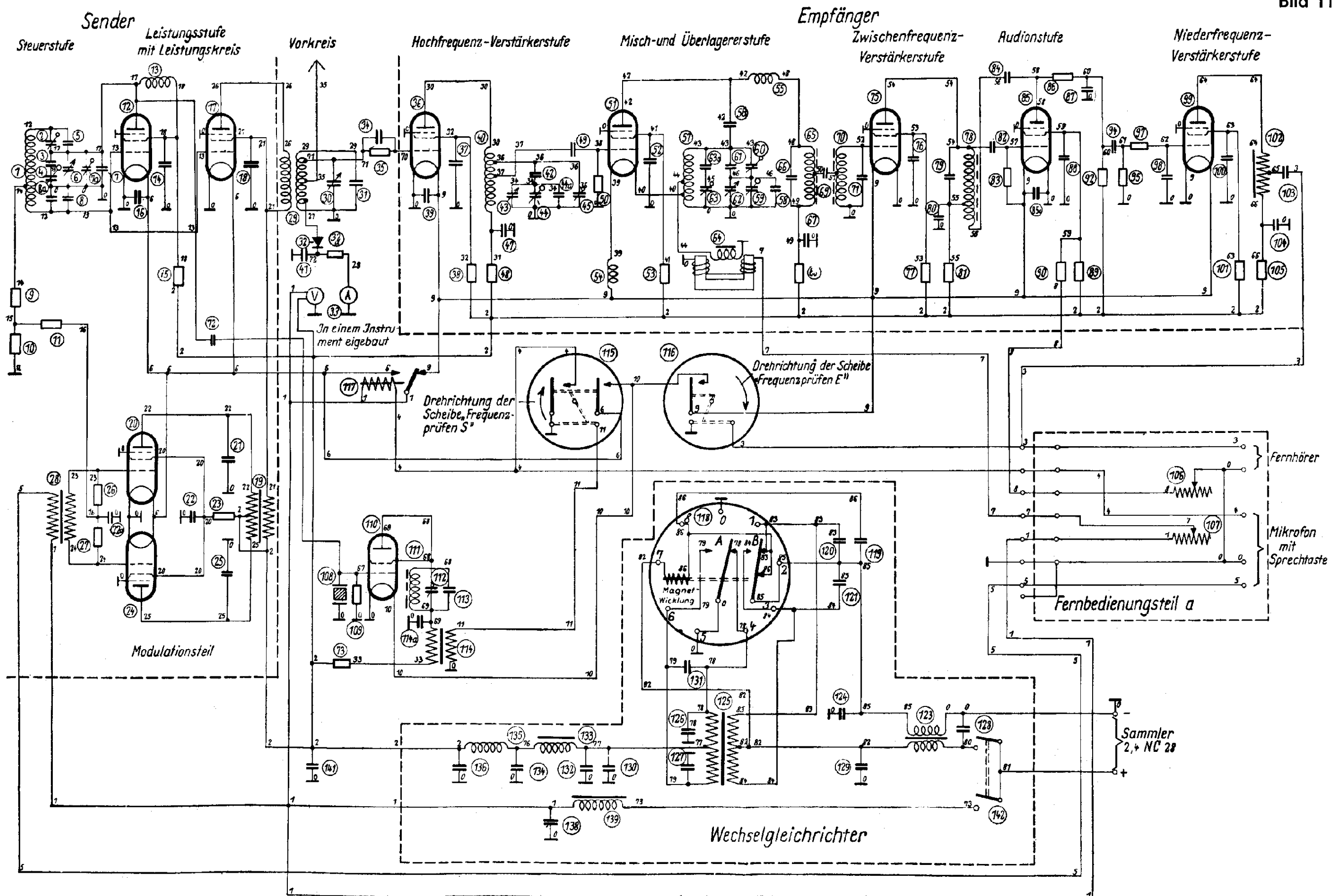
Tornisterfunkgerät h Vollständiges Schaltbild
